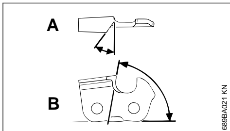
A 上刃目立て角度
